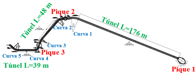
Figura 14. Vista en planta del proyecto completo.
