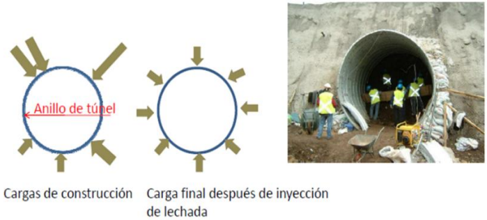
Figura 8. Ilustración de cómo la inyección de lechada entre el Tunnel liner y el suelo genera una presión uniforme.
