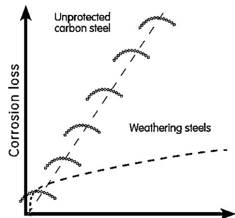
Figura 8. Comparación de pérdida de corrosión de aceros corten (weathering) con acero estructural sin protección. (Fuente: ArcelorMittal).
