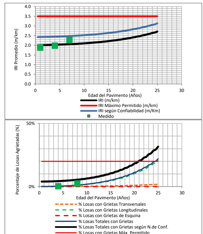
Figura 14. Resultados de desempeño medido Ruta 5 tramo Quellón — Colonia Yungay
