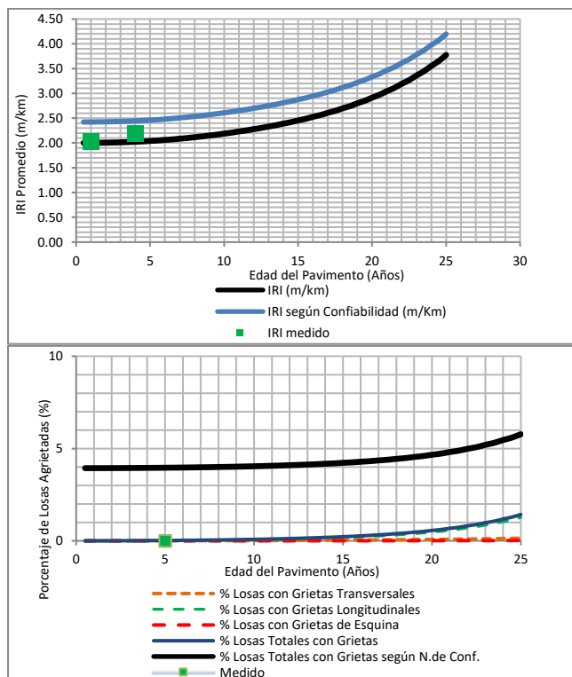
Figura 13. Resultados de desempeño medido en Ruta 60 Ch Camino La Pólvora.
