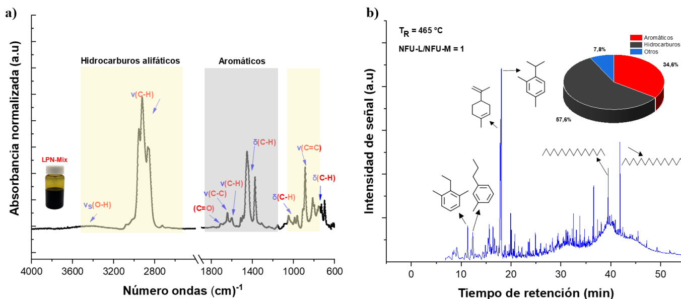
Figura 2. (a) Grupos funcionales en el LPN-Mix y determinados por FTIR-ATR; (b) Cromatograma por GC/MS del LPN-Mix que incluye la distribución de productos por grupos funcionales.
