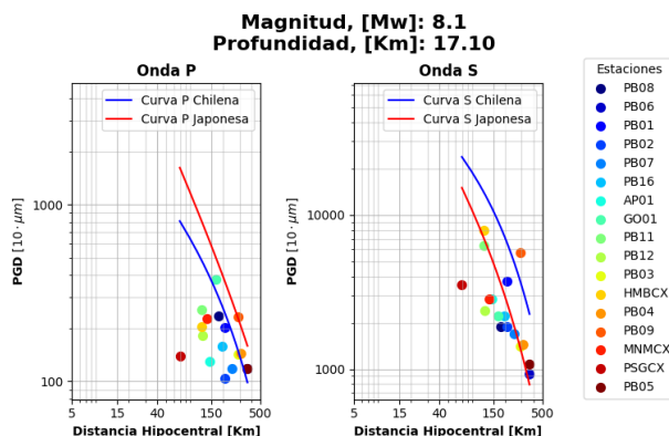
Figura 12 GMPEs Chile/Japón para 8,1Mw a 17,1 Km con un error interevento onda P de -0,139080 y onda S -0,344131 (Fuente: edición propia).
