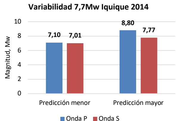
Figura 13 Variabilidad predicción magnitud de momento para evento 7,7Mw a 12 Km (Fuente: edición propia).
