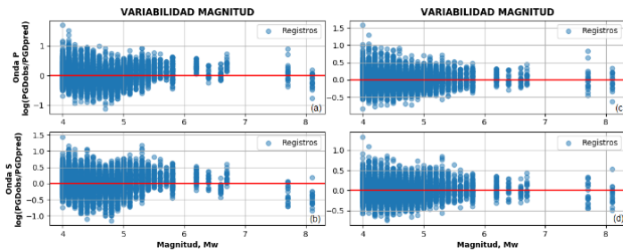
Figura 8 Variabilidad de los residuales en función de la magnitud, Mw del gap sísmico 1. (a) Residual sin ajuste onda P; (b) Residual sin ajuste onda S; (c) Residual con ajuste onda P; (d) Residual con ajuste onda S (Fuente: edición propia).
