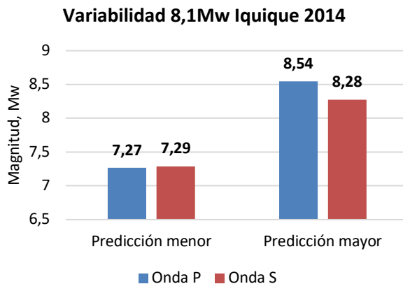
Figura 14 Variabilidad predicción magnitud de momento para evento 8,1Mw a 17,1 Km (Fuente: edición propia).
