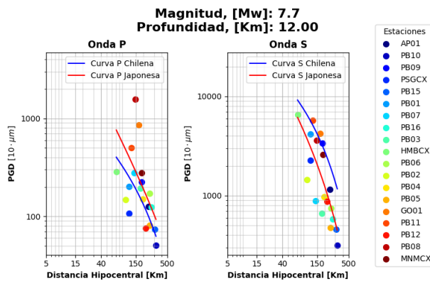
Figura 11 GMPEs Chile/Japón para 7,7Mw a 12 Km con un error interevento onda P de 0,081665 y onda S -0,261241 (Fuente: edición propia).
