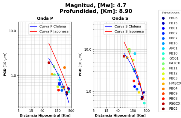
Figura 10 GMPEs Chile/Japón para 4,7Mw a 8,9 Km con un error interevento onda P de -0,024492 y onda S de -0,010953 (Fuente: edición propia).
