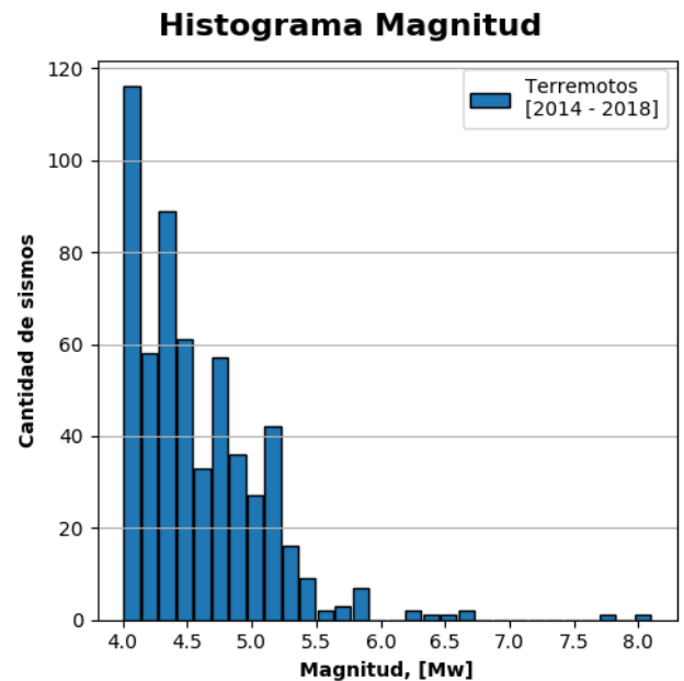
Figura 6 Histograma magnitud en base a la frecuencia de ocurrencia de eventos sísmicos y la magnitud de la actividad sísmica relacionándose con la ley de Gutenberg-Richter. En el eje x se posicionan las magnitudes de momento y en el eje y la cantidad de sismos. Las barras azules corresponden a terremotos adquiridos desde el año 2014 al 2018 los cuales están distribuidos mayoritariamente entre 4,0 Mw y 5,5 Mw. Existen solo dos terremotos de grandes magnitudes que corresponden al de Iquique de 8,2 Mw y la réplica de 7,6 Mw. Los demás sismos no sobrepasan los 7,0 Mw (Fuente: edición propia).
