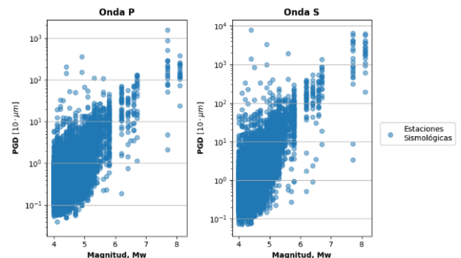
Figura 9 \log(PGD) v/s Magnitud de momento para onda P y S (Fuente: edición propia).
