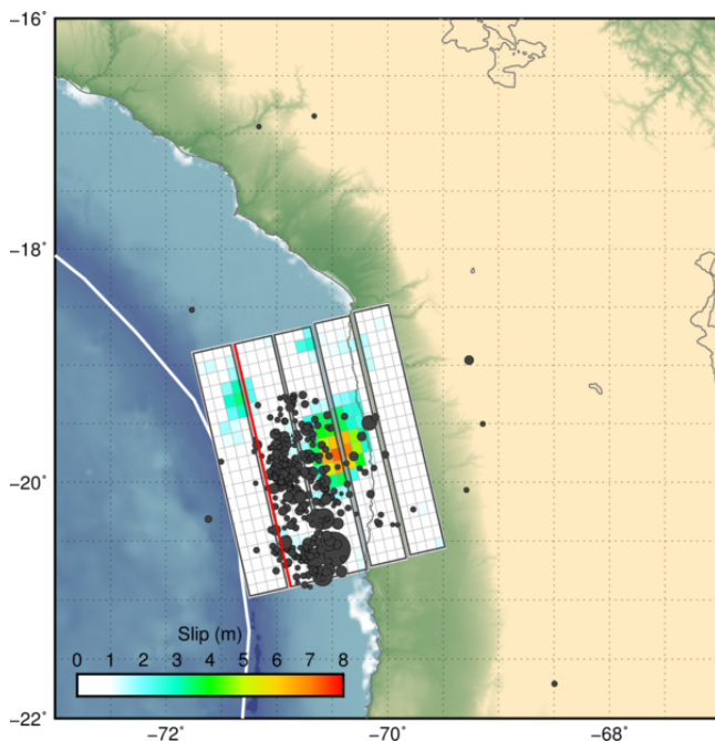
Figura 1 Modelación falla finita terremoto 8,2 Mw Iquique 2014 (Fuente: extraído de (United States Geological Survey (USGS), 2018)).
