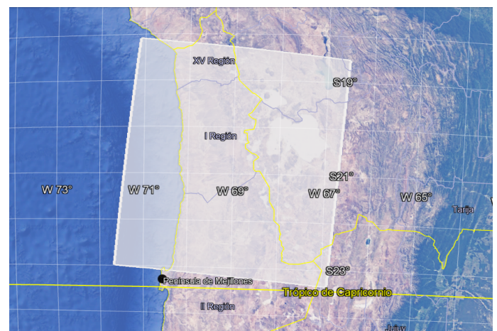
Figura 3 Gap sísmico norte de Chile (Fuente: edición propia)
